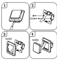
Obrázok 2. Demontáž termostatu
