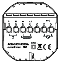
Obrázok 1. Popis svorkovnice termostatu
